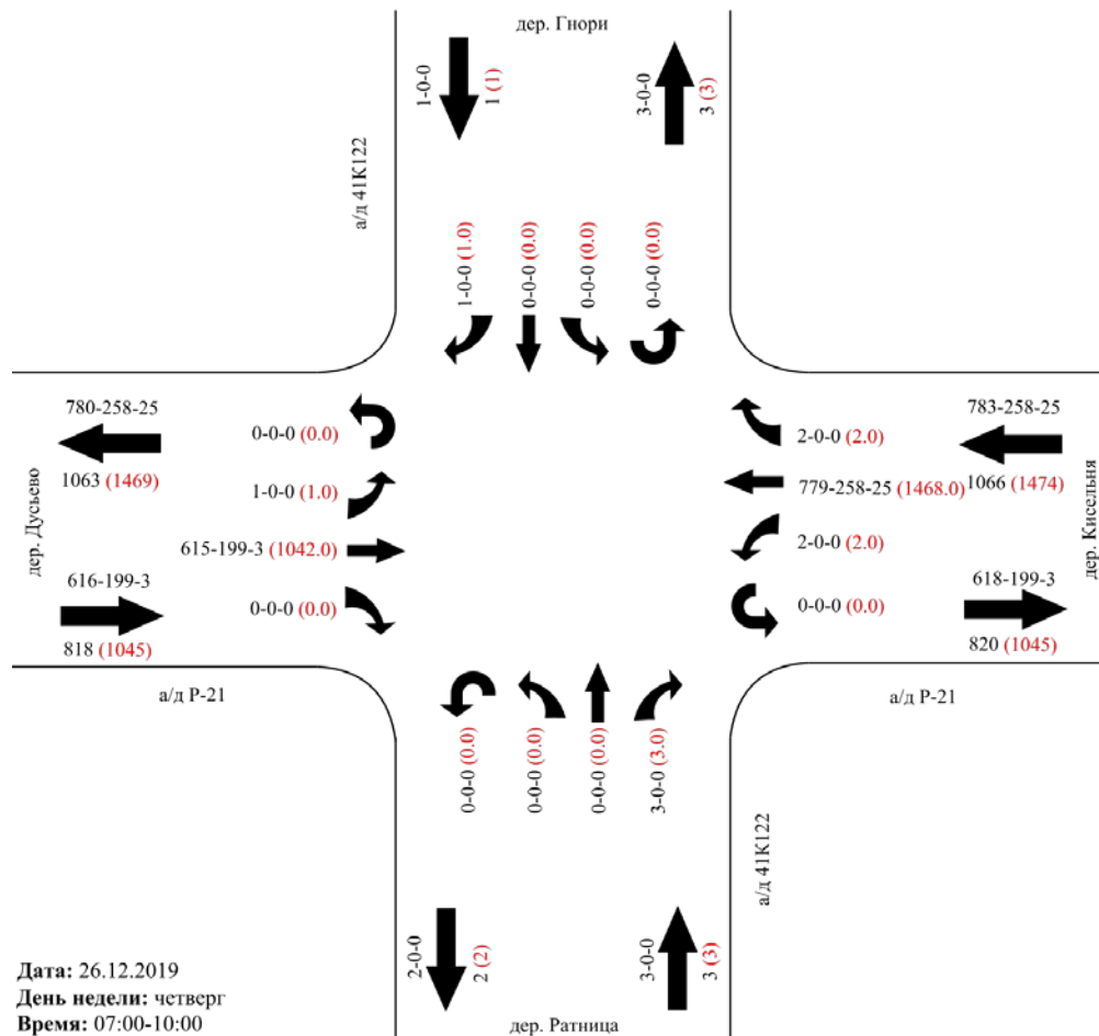
Картограмма интенсивности участка № 5 Участок/перекресток: а/д Р-21 - а/д 41К122 (Ратница)
