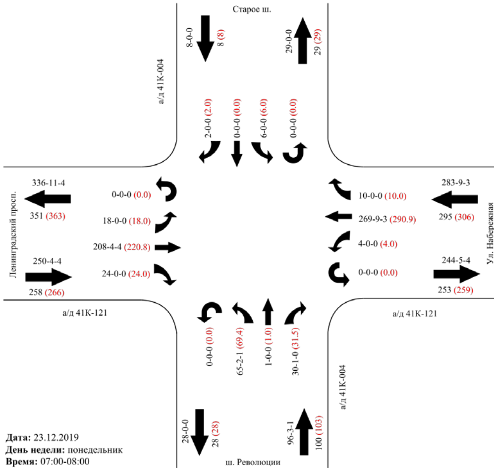
Картограмма интенсивности участка № 12 Участок/перекресток: а/д 41К-121 – а/д 41К-004
