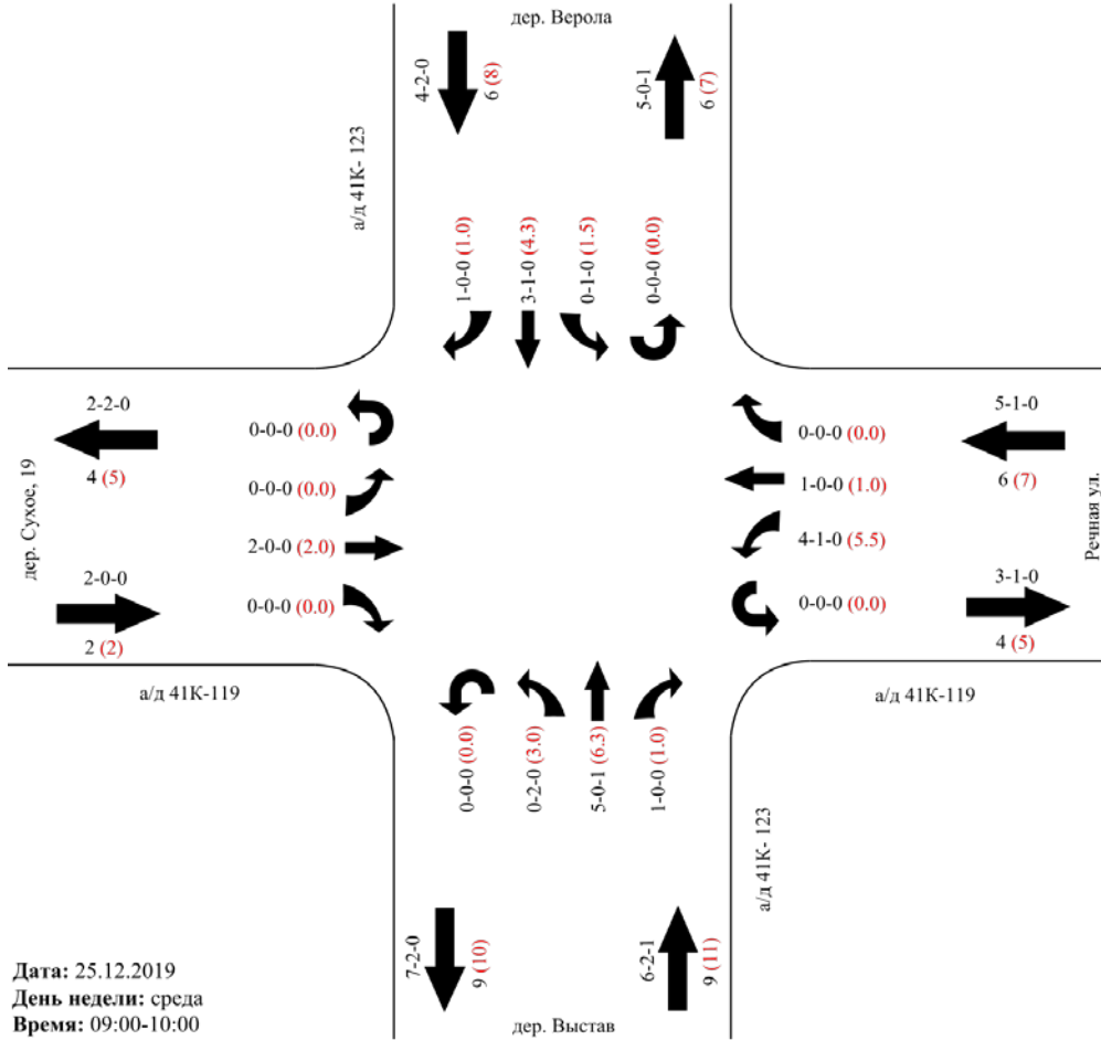
Картограмма интенсивности участка № 13 Участок/перекресток: а/д 41К-123 – а/д 41К-119
