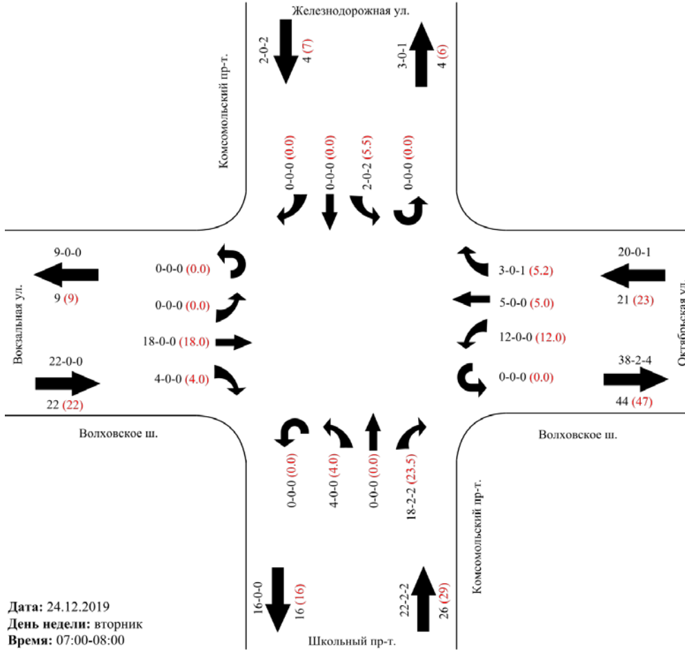
Картограмма интенсивности участка № 19 Участок/перекресток: Городской поселок Назия, Волховское ш. – Комсомольский пр-т.
