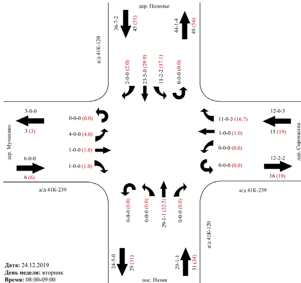
Картограмма интенсивности участка № 3 Участок/перекресток: а/д 41К-239 - а/д 41К-120
