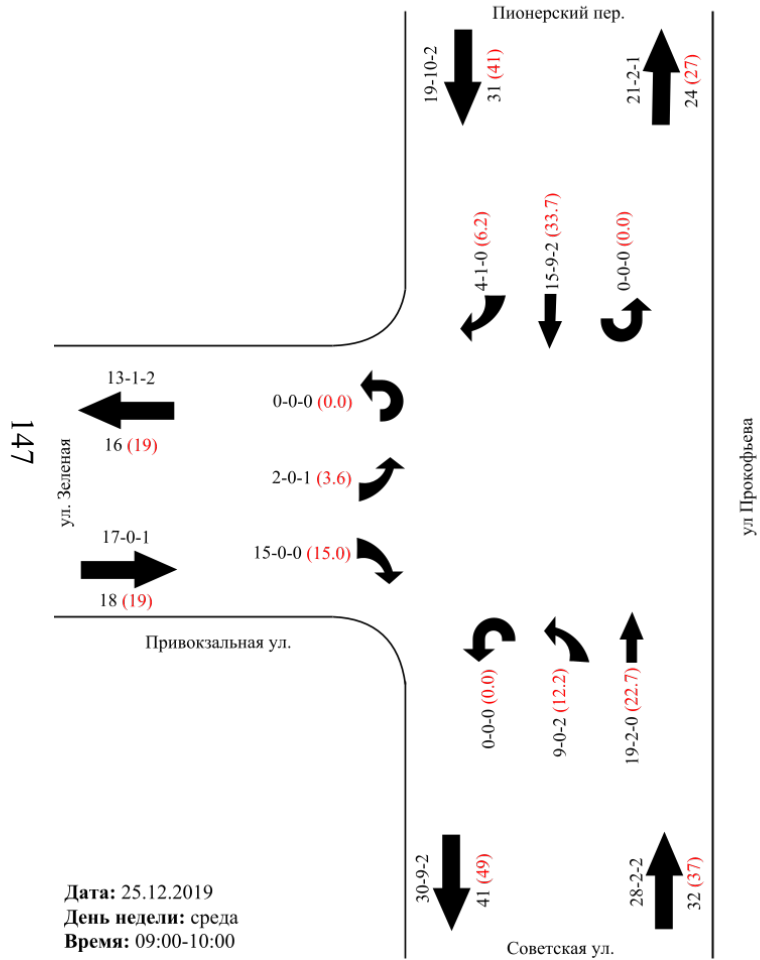
Картограмма интенсивности участка № 6 Участок/перекресток: ул. Прокофьева - Привокзальная ул.
