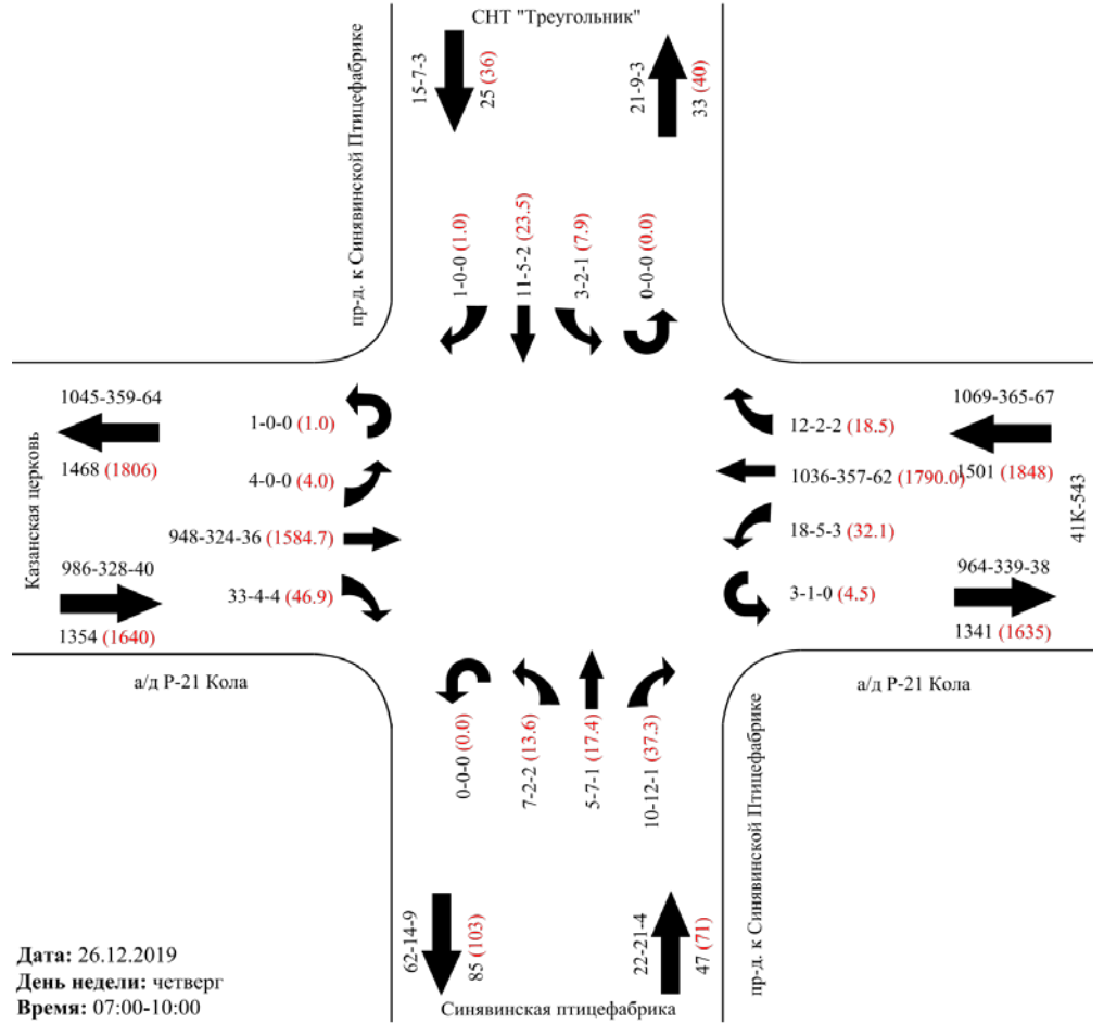
Картограмма интенсивности участка № 16 Участок/перекресток: а/д Р-21 – проезд к Синявинской Птицефабрике
