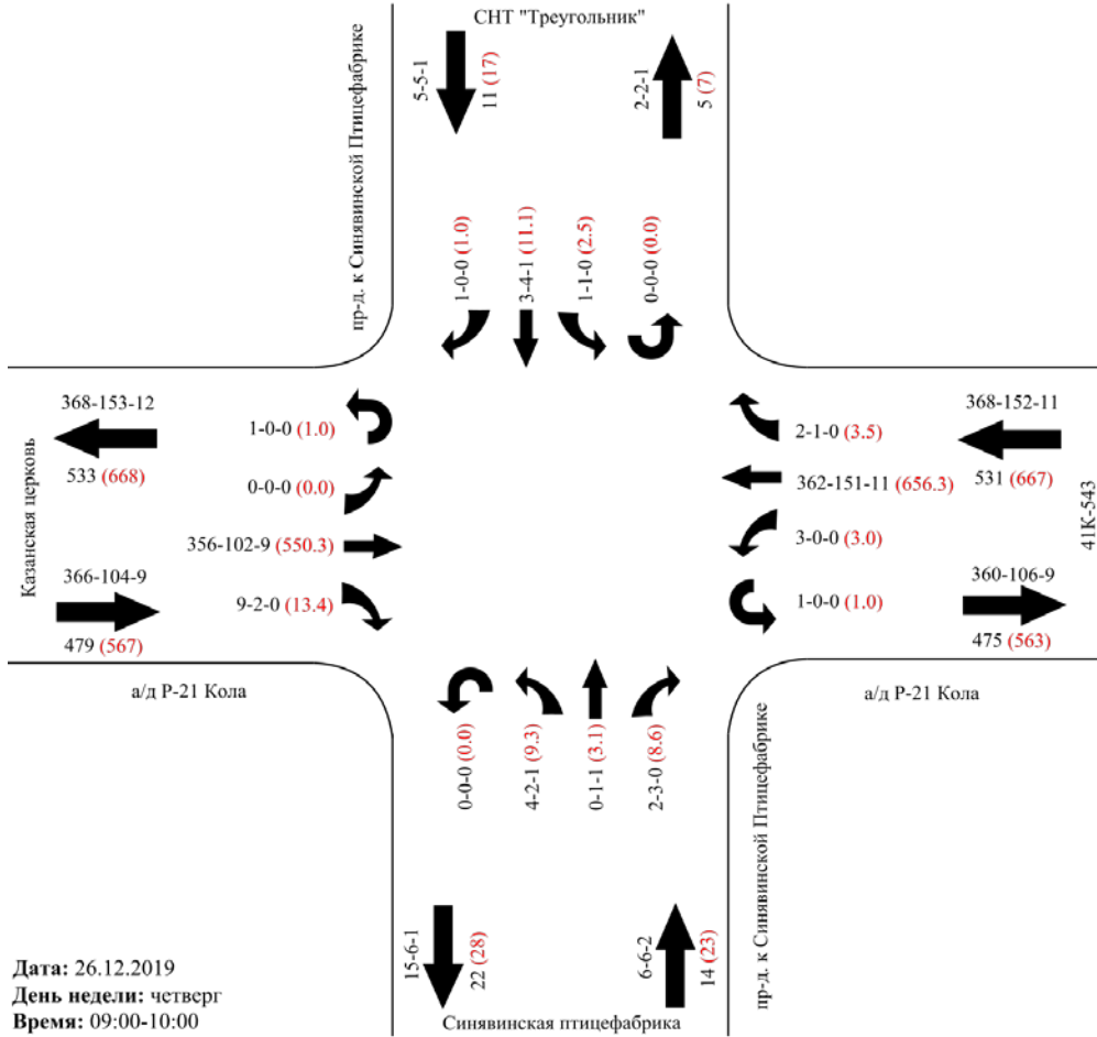
Картограмма интенсивности участка № 16 Участок/перекресток: а/д Р-21 – проезд к Синявинской Птицефабрике
