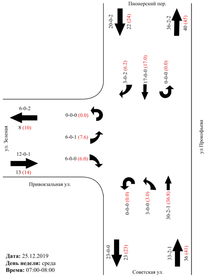
Картограмма интенсивности участка № 6 Участок/перекресток: ул. Прокофьева - Привокзальная ул.
