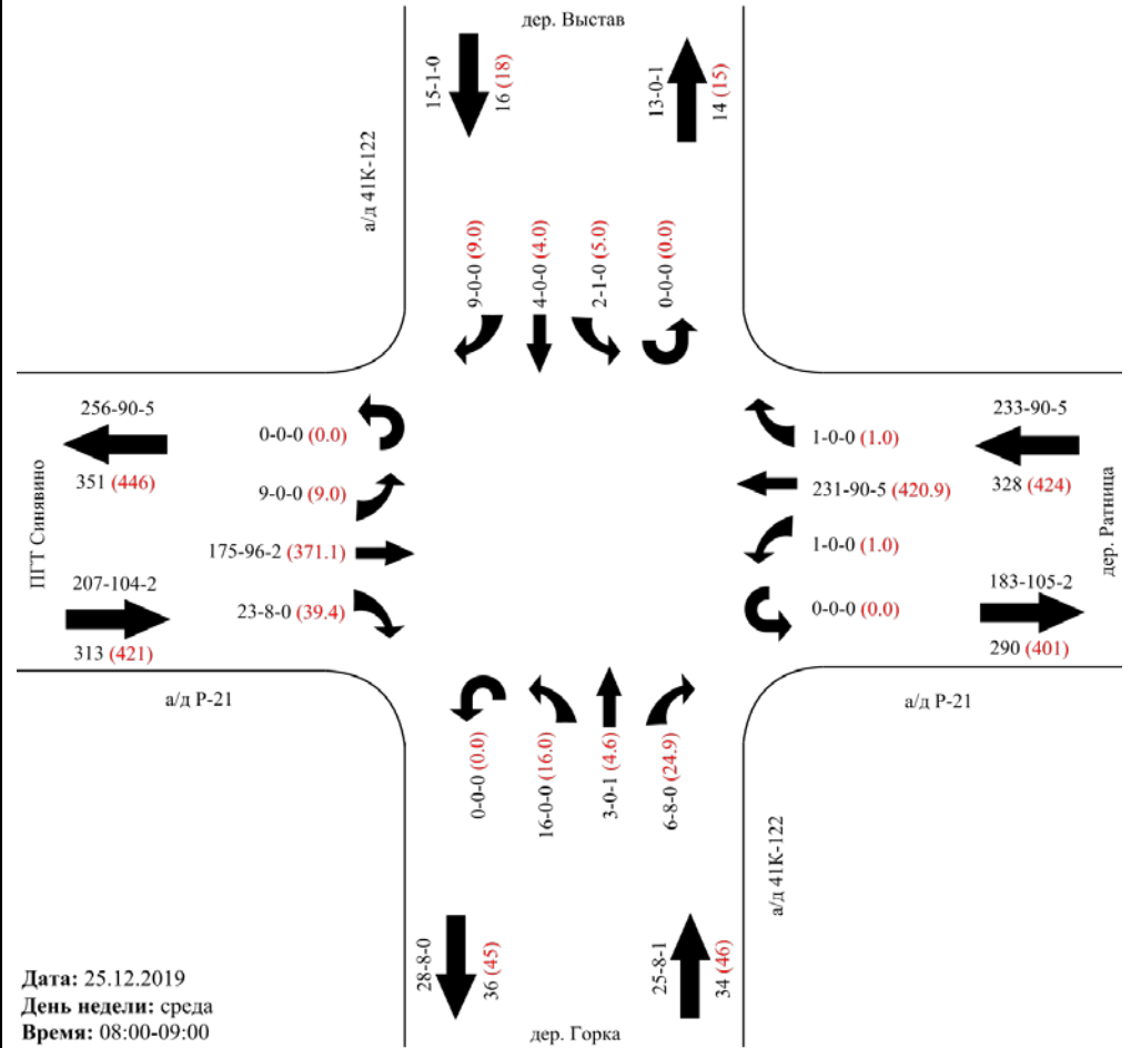
Картограмма интенсивности участка № 4 Участок/перекресток: а/д Р-21 - а/д Р-21
