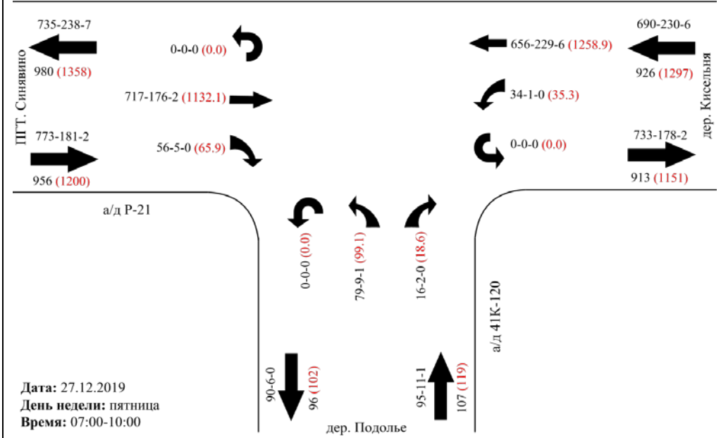
Картограмма интенсивности участка № 2 Участок/перекресток: а/д Р-21 - а/д 41К-120
