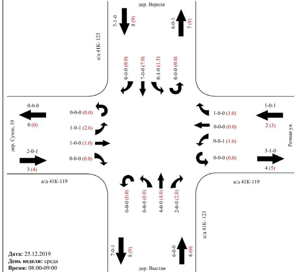
Картограмма интенсивности участка № 13 Участок/перекресток: а/д 41К-123 – а/д 41К-119
