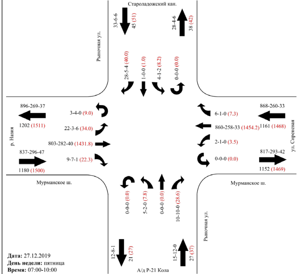
Картограмма интенсивности участка № 8 Участок/перекресток: а/д Р-21 – Рыночная ул. поворот на Назию
