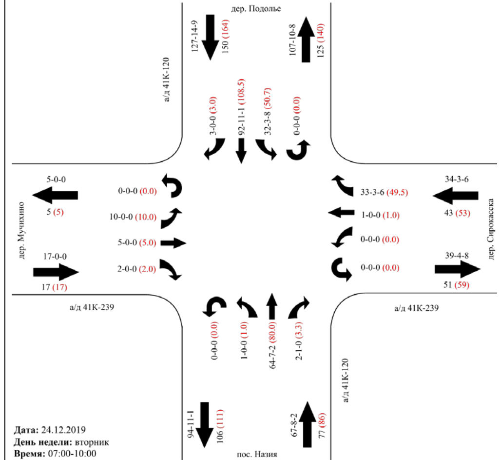
Картограмма интенсивности участка № 3 Участок/перекресток: а/д 41К-239 - а/д 41К-120
