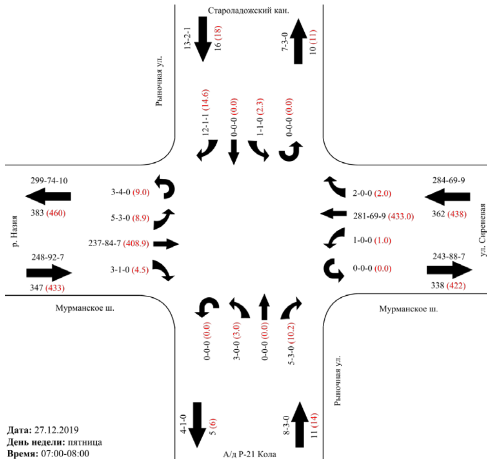
Картограмма интенсивности участка № 8 Участок/перекресток: а/д Р-21 – Рыночная ул. поворот на Назию
