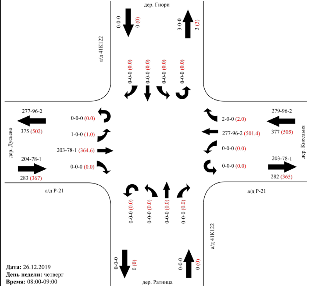
Картограмма интенсивности участка № 5 Участок/перекресток: а/д Р-21 - а/д 41К122 (Ратница)
