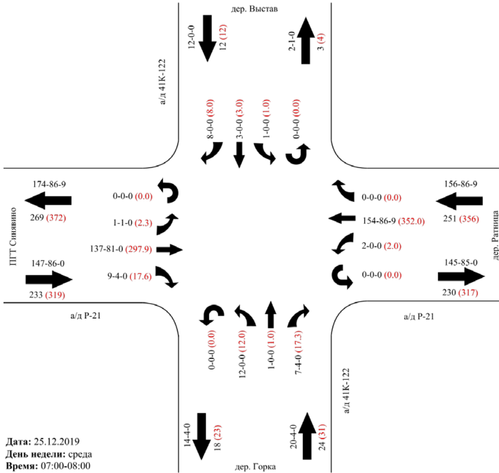
Картограмма интенсивности участка № 4 Участок/перекресток: а/д Р-21 - а/д Р-21
