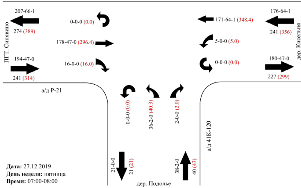
Картограмма интенсивности участка № 2 Участок/перекресток: а/д Р-21 - а/д 41К-120
