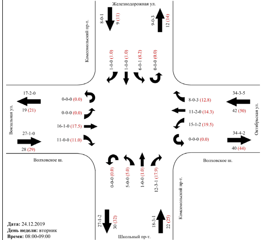
Картограмма интенсивности участка № 19 Участок/перекресток: Городской поселок Назия, Волховское ш. – Комсомольский пр-т.
